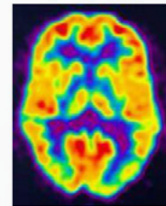
^{18}\text{F} -FDG
