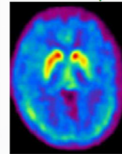
^{18}\text{F} -FDG
