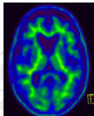
^{18}\text{F} -Estirilpiridina
